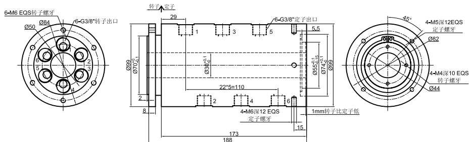
GJ6030-04 外形尺寸图
